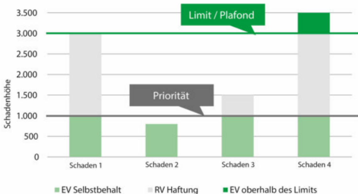
Abbildung 4.8: Funktionsweise des Einzelschadenexzedenten
