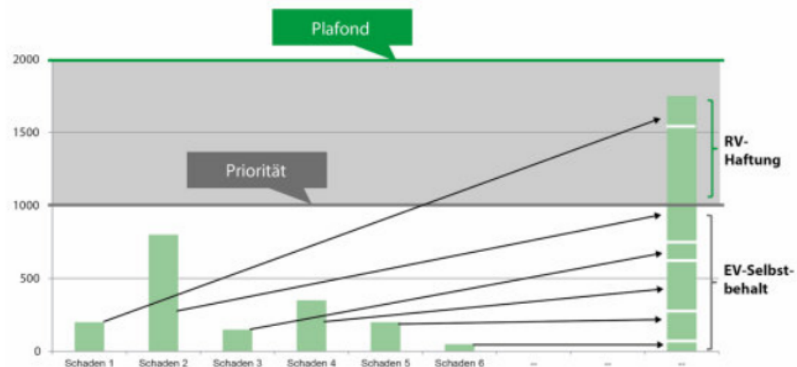
Abbildung 4.9: Beispiel Cat-XL (1.000 xs. 1.000) mit Schäden aus einem Kumulereignis
